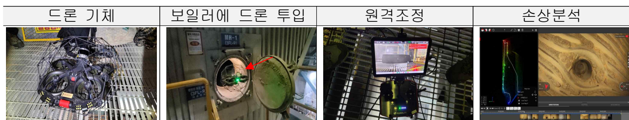
[그림 2] 드론을 이용한 보일러 내부점검 사진
